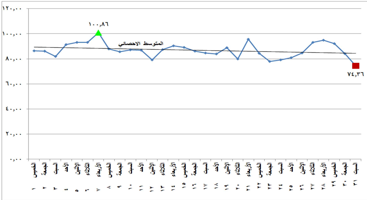
شكل (٢١) الطاقة الكهربائية المنتجة من المصادر غير الحرارية خلال شهر يوليو ٢٠٢١
