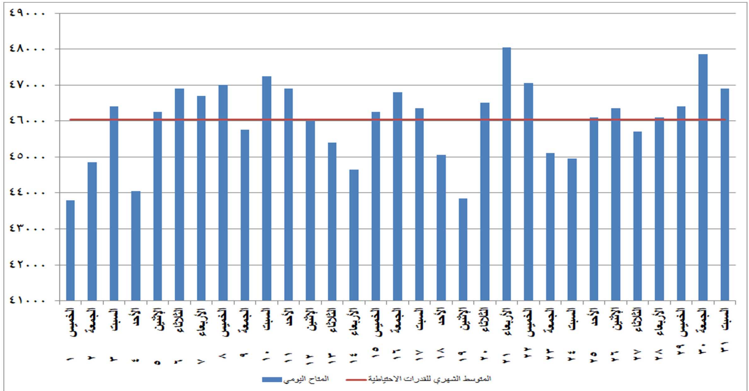
شكل (٢٧) القدرات المتاحة يوميا والمتوسط الشهري للقدرة الاحتياطية خلال شهر يوليو ٢٠٢١
