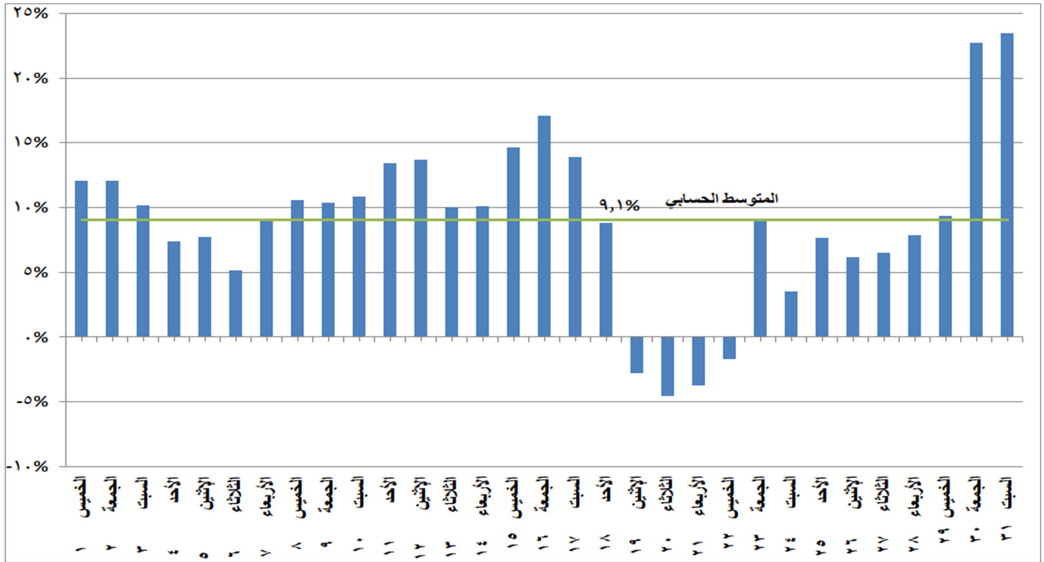
شكل (٩) النسب المئوية للتغير في الحمل الاقصى خلال شهر ٢٠٢١ مقارنة باليوم المماثل من العام الماضي
