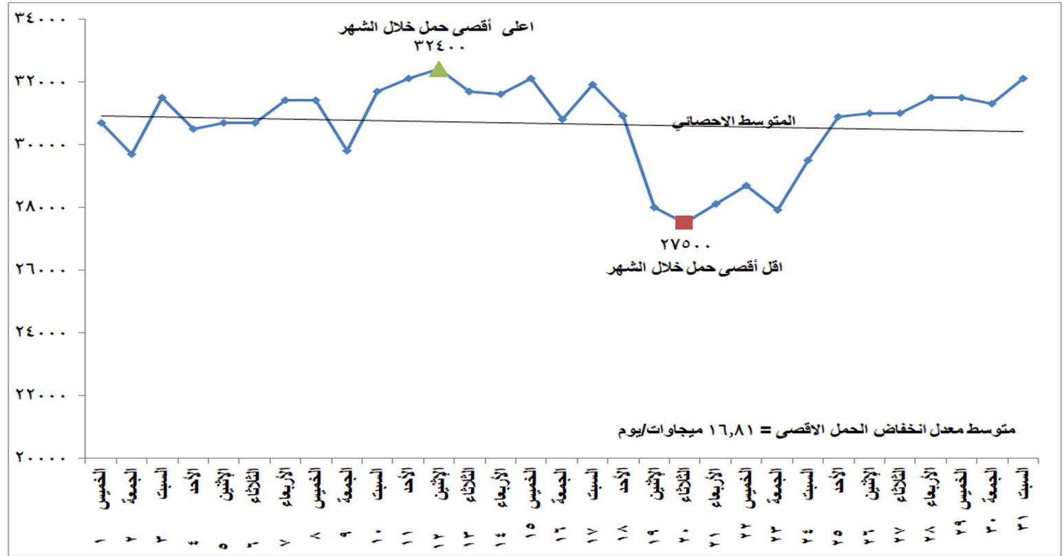
شكل (١) تطور الحمل الاقصى اليومي خلال شهر يوليو ٢٠٢١
