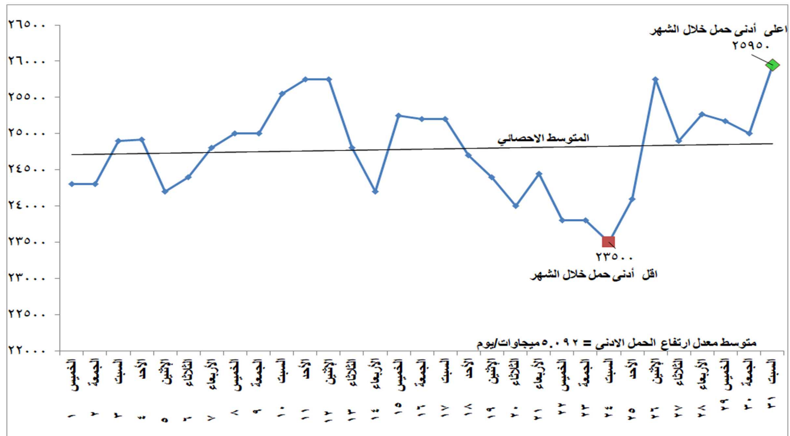
شكل (٢) تطور الحمل الادنى اليومي خلال شهر يوليو ٢٠٢١
