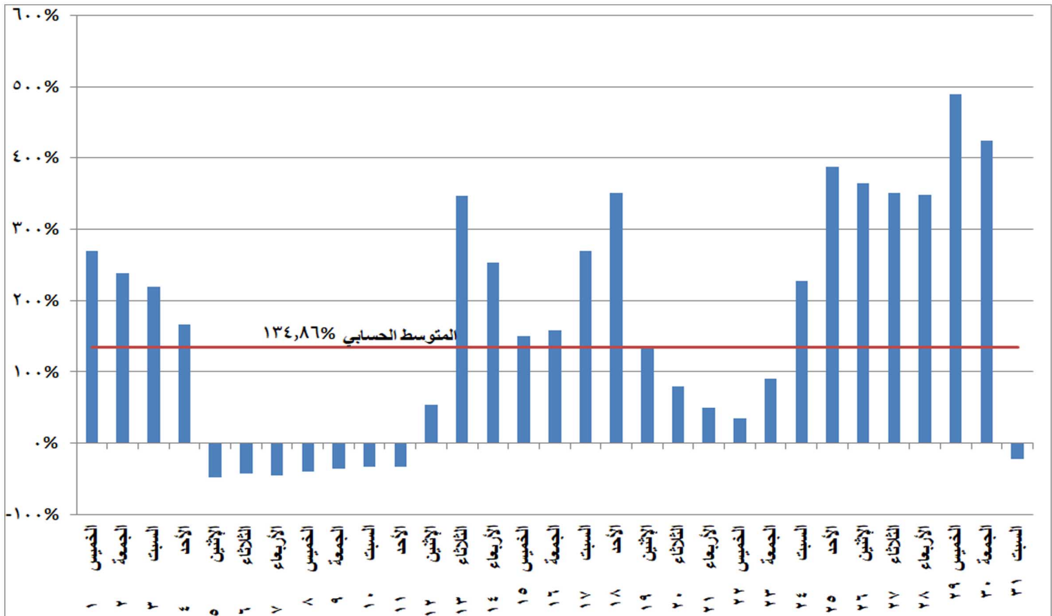
شكل (٢٠) نسب التغير في استخدام المازوت في إنتاج الطاقة الكهربائية خلال شهر يوليو ٢٠٢١ مقارنة بالشهر المماثل من العام السابق
