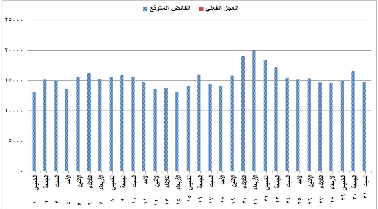
شكل (٧) الفاضل والعجز المتوقع للقدرات خلال شهر يوليو ٢٠٢١
