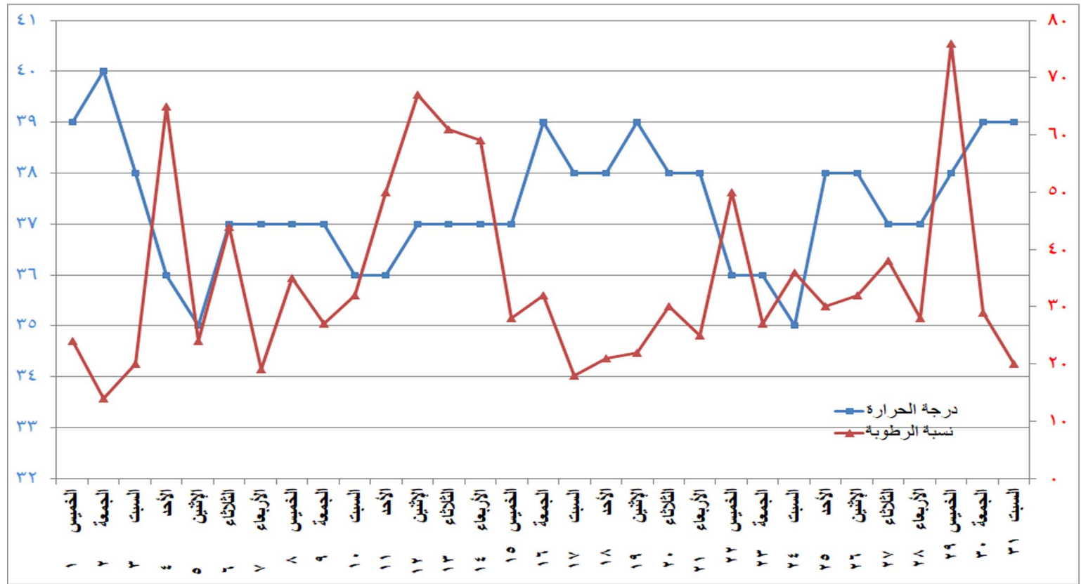
شكل (١١) التغيير في درجة الحرارة والرطوبة النسبية خلال شهر يوليو ٢٠٢١
