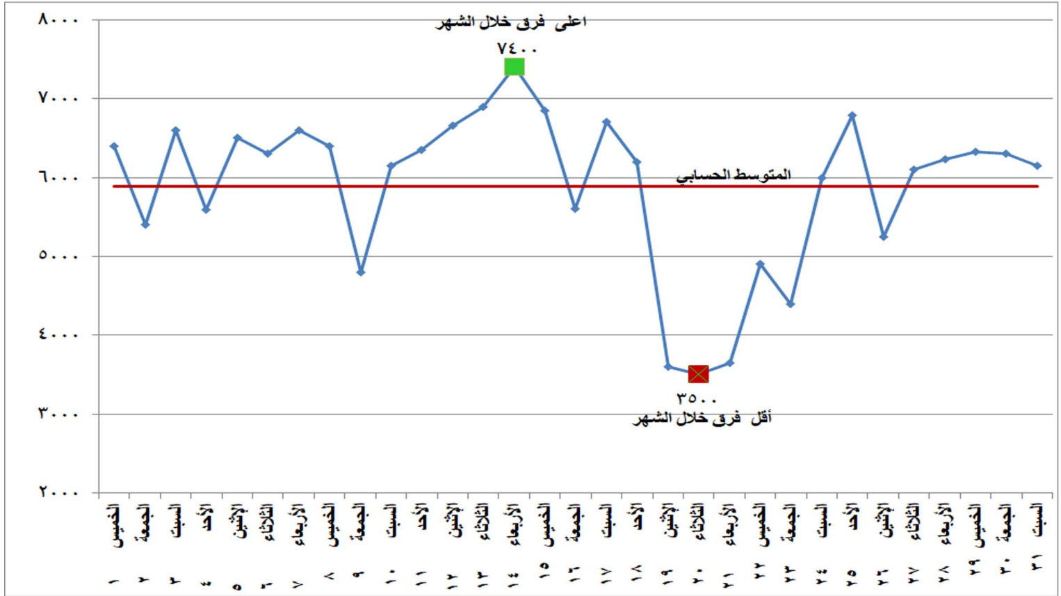
شكل (٣) الفرق بين أقصى وأدنى حمل خلال شهر يوليو ٢٠٢١
