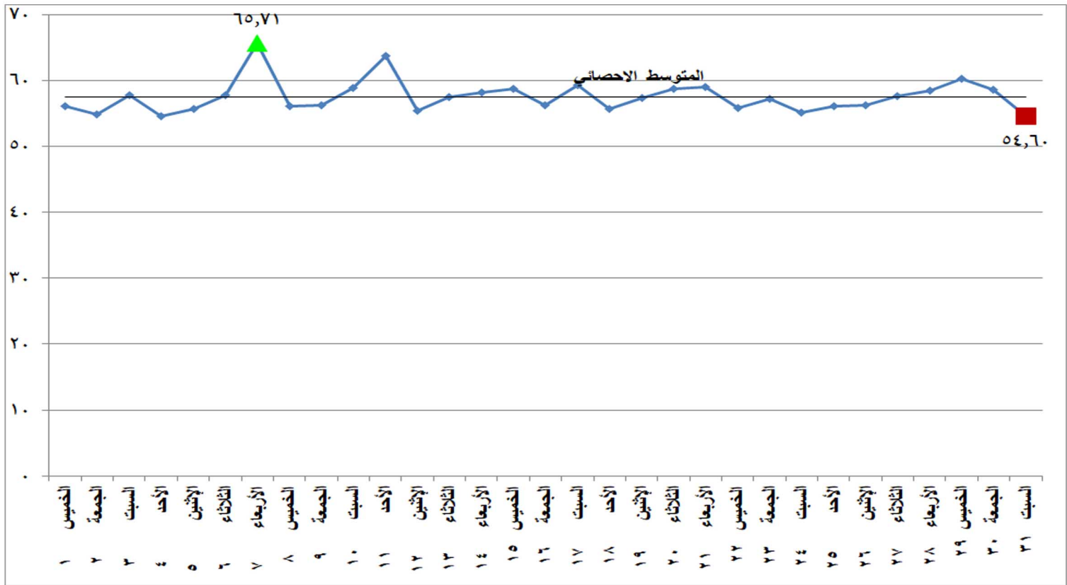
شكل (٢٣) الطاقة الكهربائية المنتجة من المصادر المائية خلال شهر يوليو ٢٠٢١
