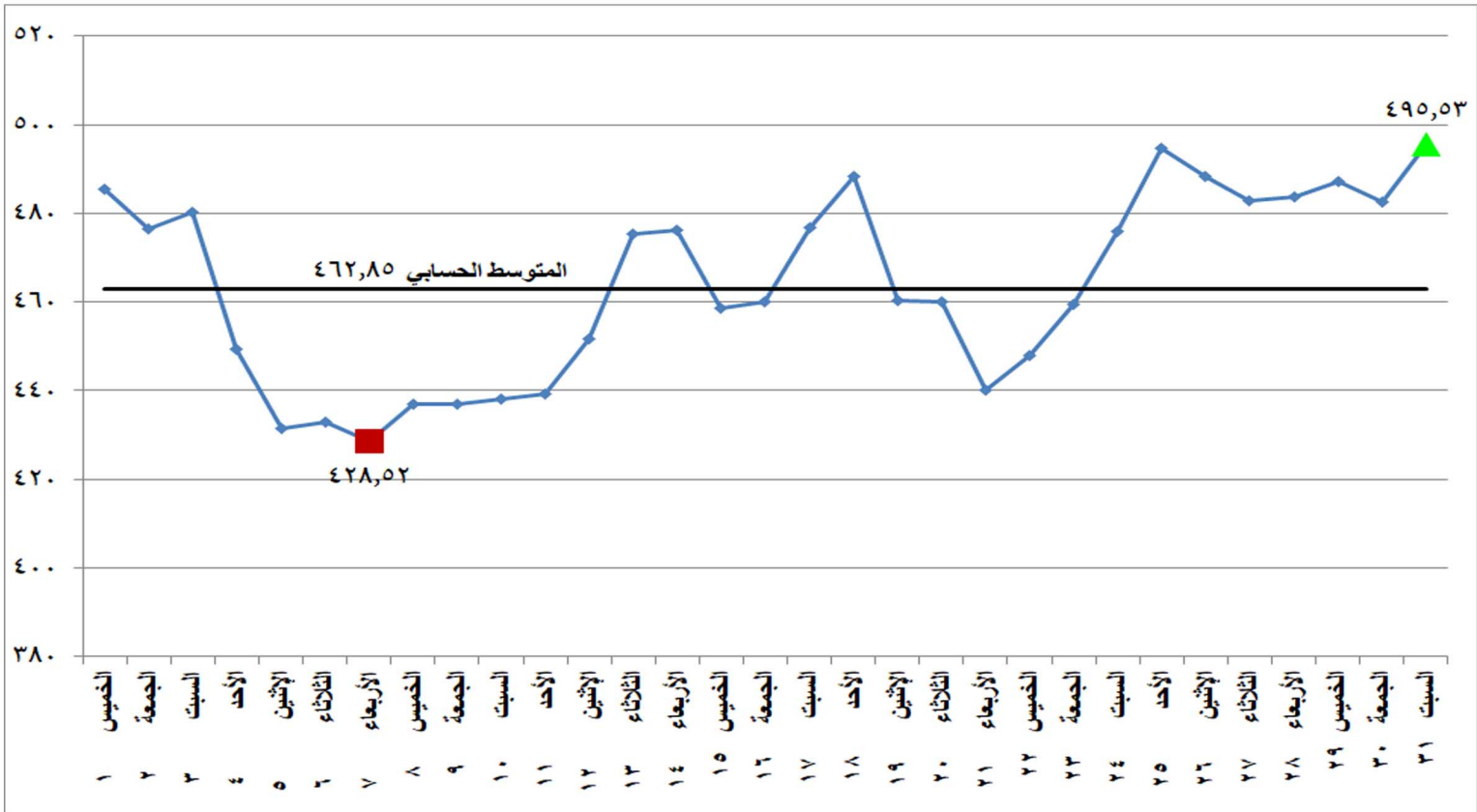
شكل (١٤) معامل انبعاثات غاز ثاني اكسيد الكربون المكافئ على مدى شهر يوليو ٢٠٢١
