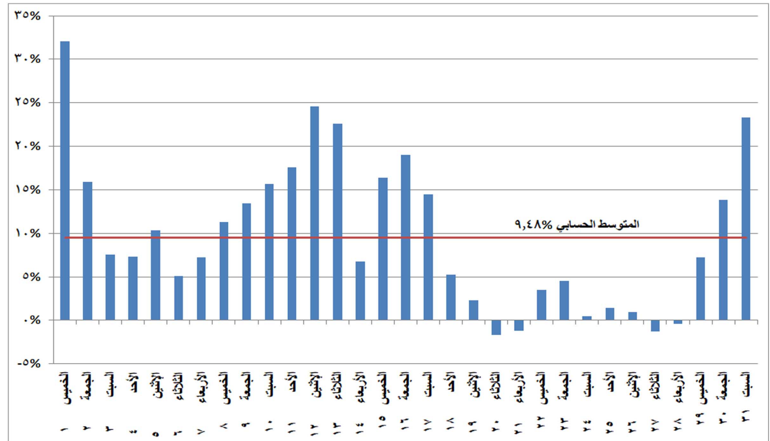
شكل (١٨) نسب التغير في استخدام الغاز الطبيعي في إنتاج الطاقة الكهربائية خلال شهر يوليو ٢٠٢١ مقارنة بالشهر المماثل من العام السابق
