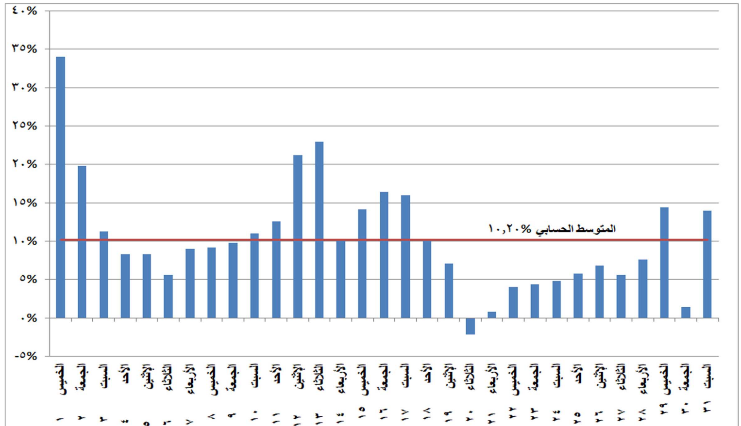
شكل (١٦) نسب التغير في الطاقة الكهربائية المنتجة خلال شهر يوليو ٢٠٢١ مقارنة بالشهر المماثل من العام السابق
