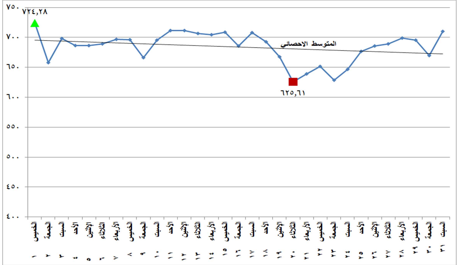
شكل (١٥) إجمالي الطاقة الكهربائية المنتجة من كل المصادر الأولية خلال شهر يوليو ٢٠٢١
