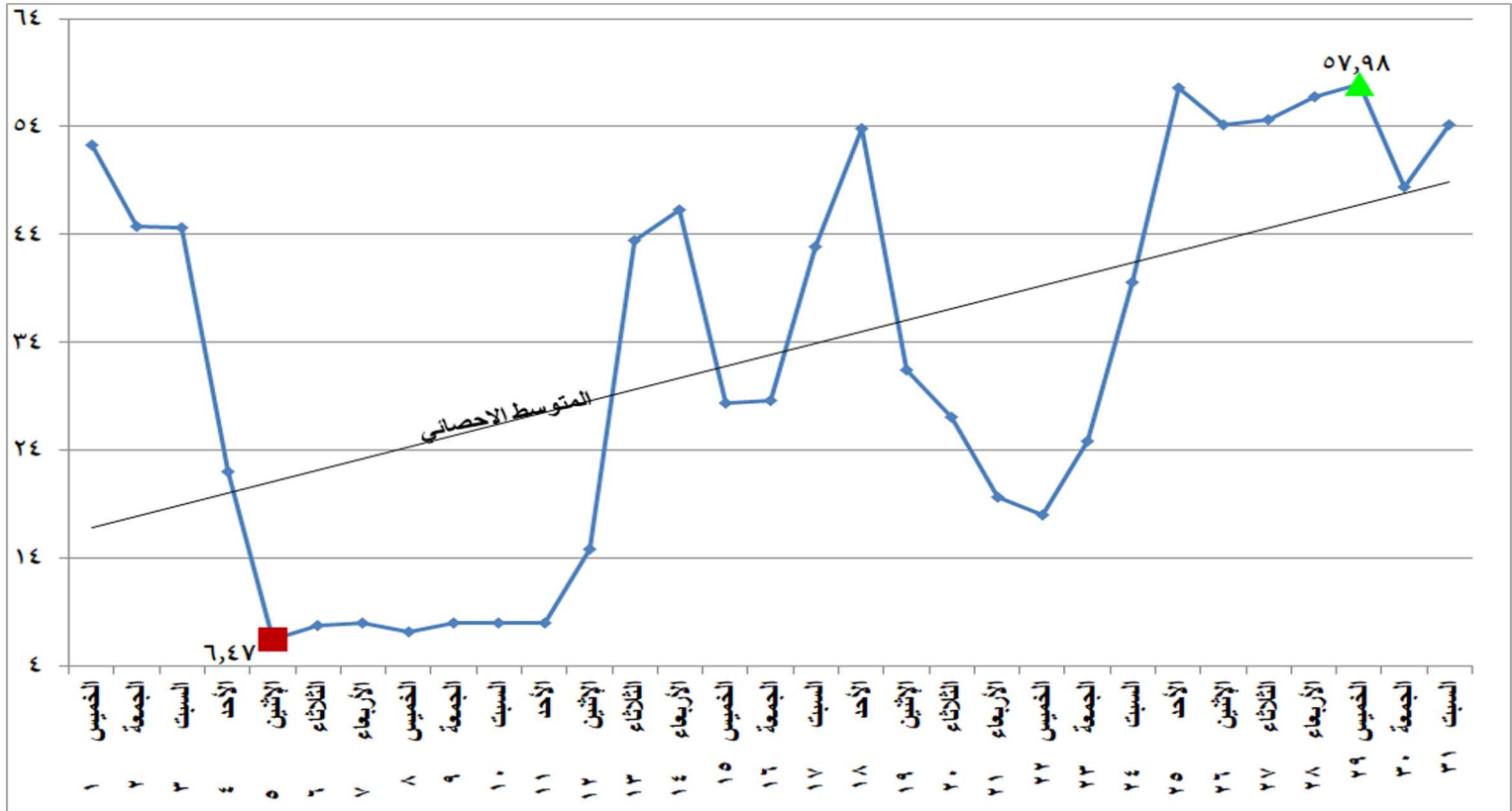
شكل (١٩) الطاقة الكهربائية المنتجة من المازوت خلال شهر يوليو ٢٠٢١
