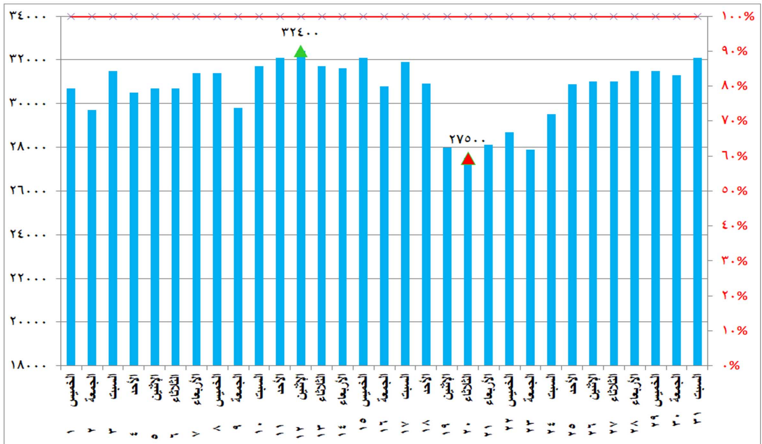
شكل (٥) قدرات الانتاج المتاحة ونسبتها للحمل الأقصى خلال شهر يوليو ٢٠٢١
