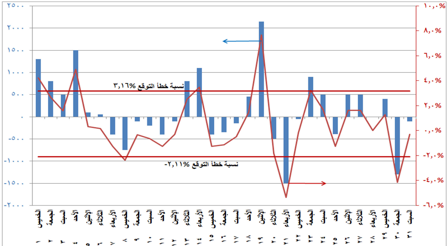
شكل (١٠) الفرق بين الحمل الأقصى المتوقع والمسجل فعليا ونسبة الفرق إلى الحمل المسجل فعليا خلال شهر يوليو ٢٠٢١
