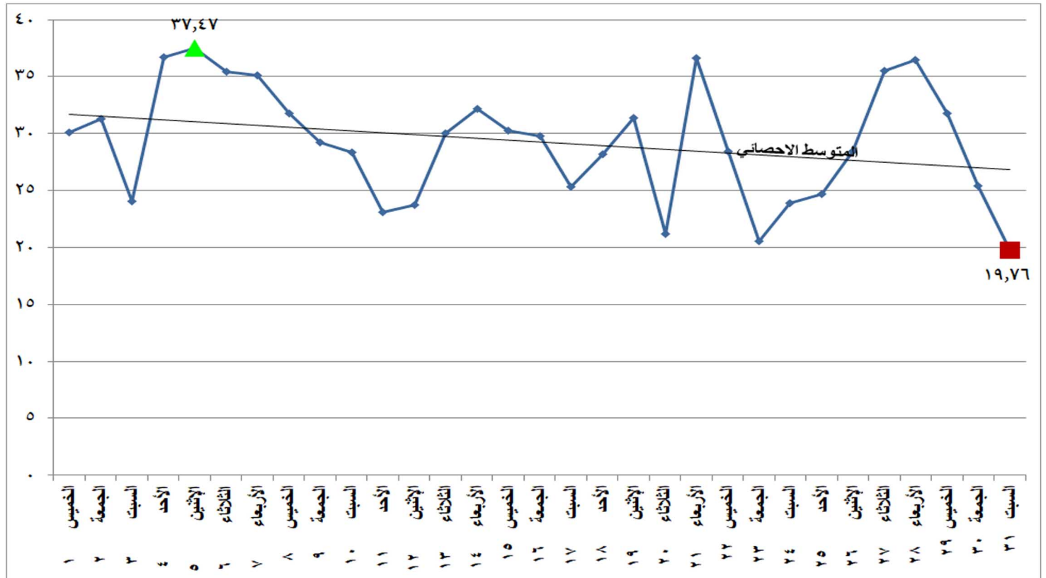
شكل (٢٥) الطاقة الكهربائية المنتجة من الرياح والشمس خلال شهر يوليو ٢٠٢١
