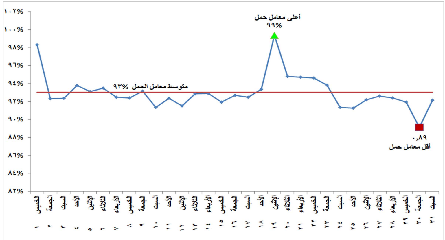
شكل (١٢) إجمالي معامل الحمل لوحدات الانتاج خلال شهر يوليو ٢٠٢١
