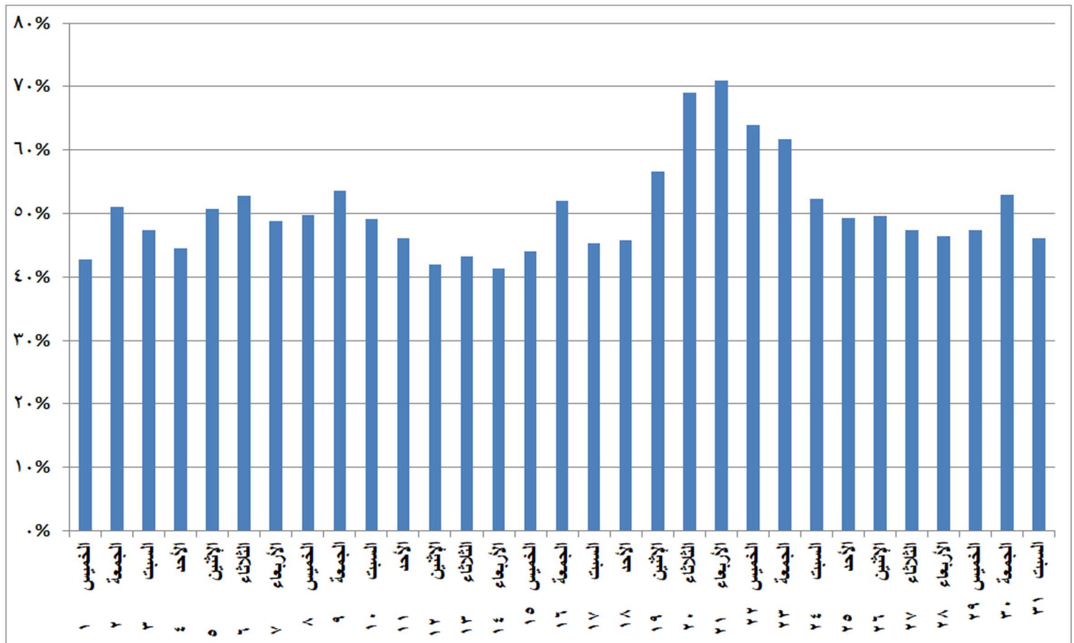
شكل (٢٨) نسب الفائض للحمل الاقصى المسجل يوميا خلال شهر يوليو ٢٠٢١
